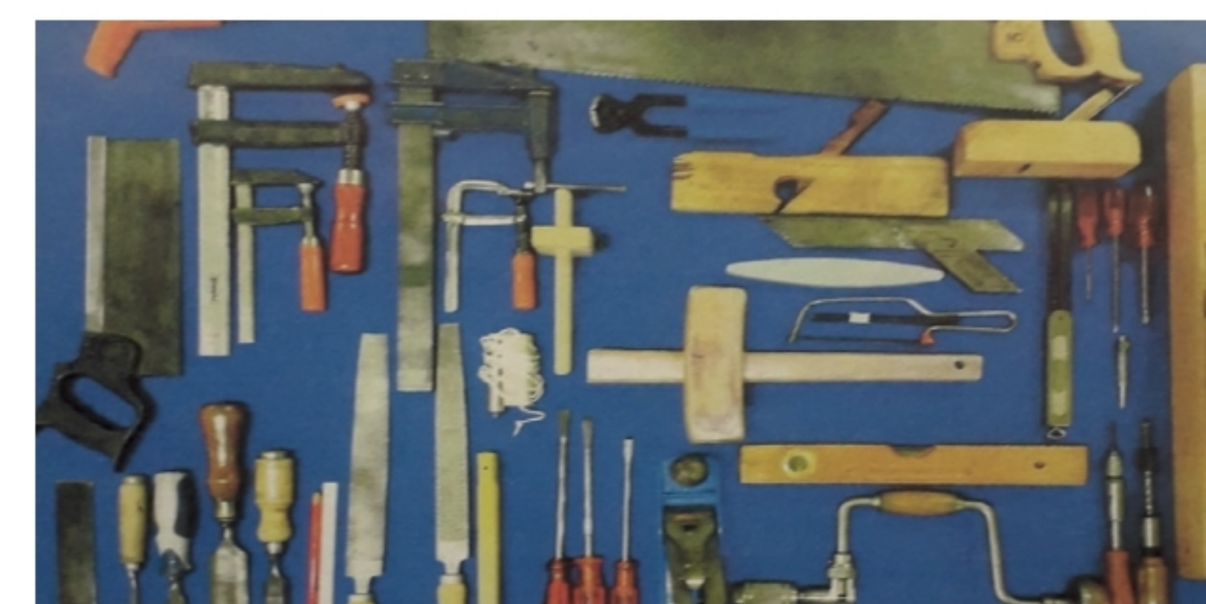
Gereedschapset timmerman
